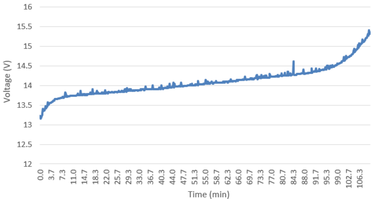
C10 2020-jan-03 17:00 Charge 12Ah battery
