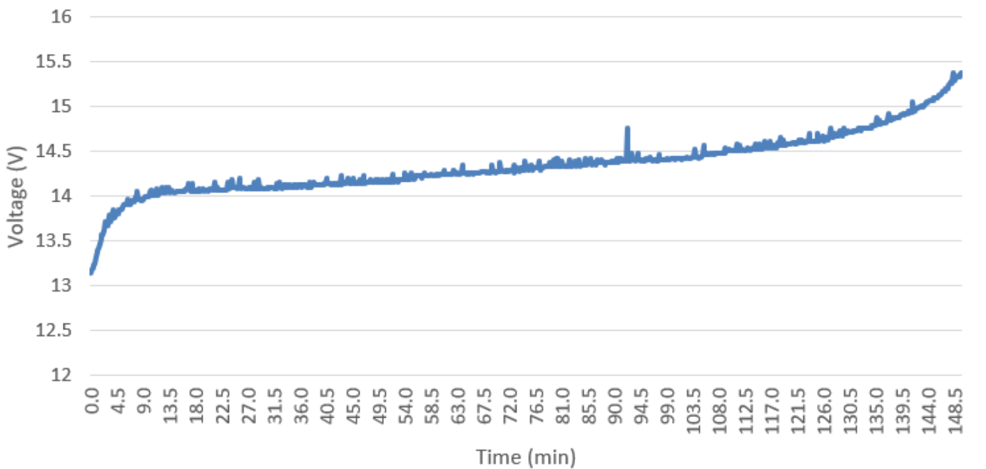
C8 2020-jan-02 08:31 Charge 12Ah battery
